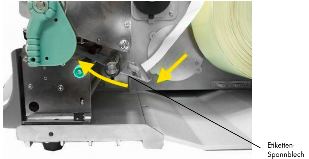
Abb. 5.2.1.i Material einlegen
