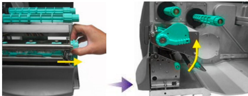
Abb. 5.3.1.a Druckkopf-Andruckhebel herausziehen und hoch schwenken (entgegen dem Uhrzeigersinn).
