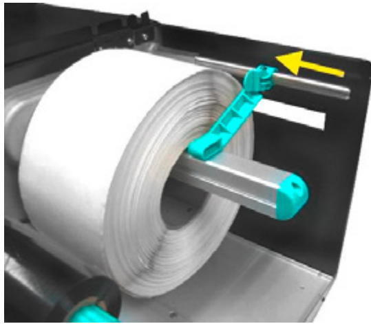
Abb. 5.2.1.g Führung Etikettenzufuhr richtig einstellen
