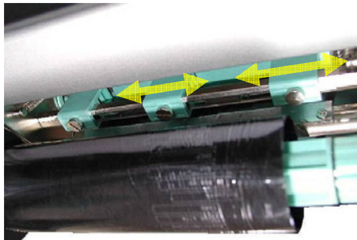
Abb. 5.4.c Druckfederboxen seitlich verschieben
