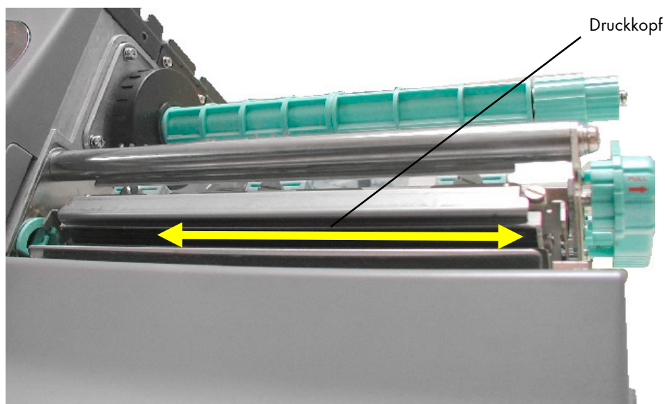
Abb. 9.1.2.a Druckkopfes reinigen
