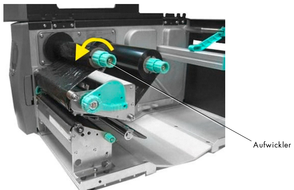
Abb. 5.3.1.e Folie durch Drehung des Farbband-Aufwicklers spannen
