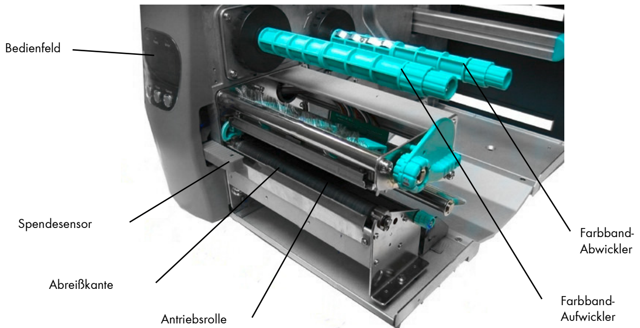
Abb. 2.4.d Detailaufnahme Druckmechanik
