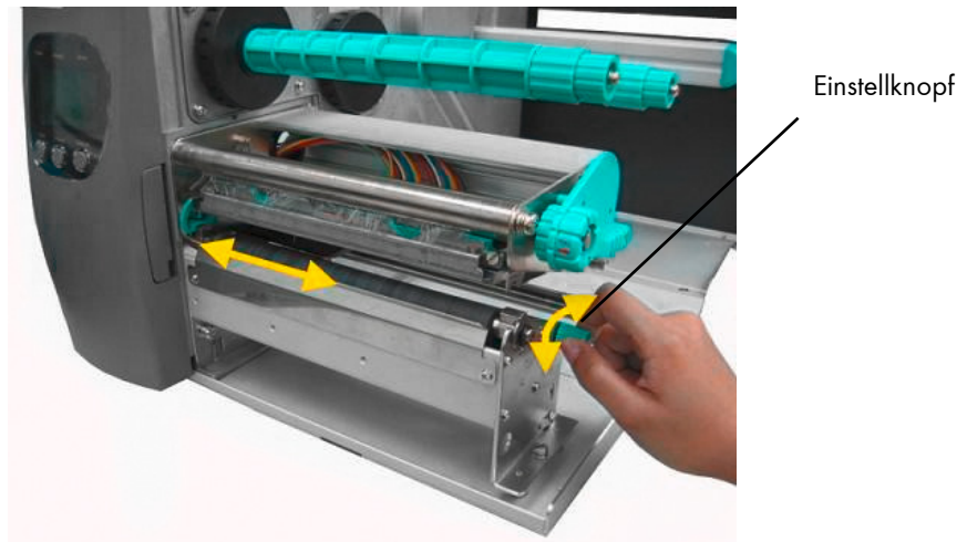
Abb. 5.2.1.k Sensorposition verstellen
