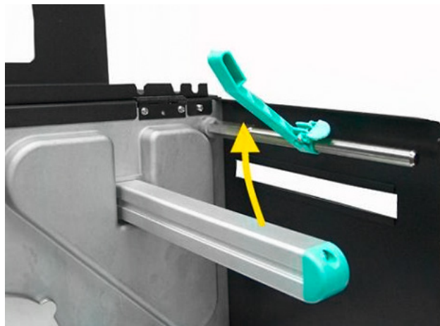
Abb. 5.2.1.d Führung Etikettenzufuhr nach oben schwenken
