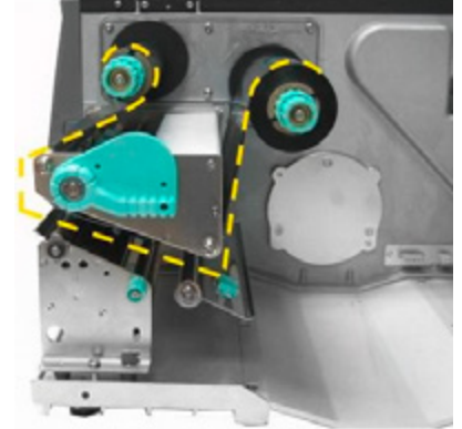
Abb. 5.3.1.b Unterschiedliche Wickelrichtungen für Folienrollen
