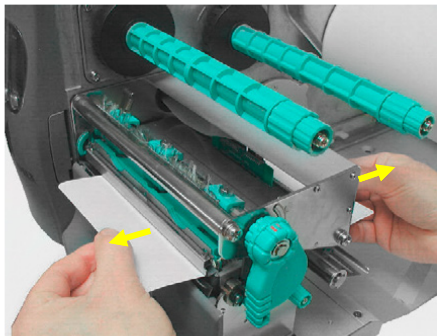
Abb. 9.1.2.c Reinigungsstreifen hin- und herbewegen
