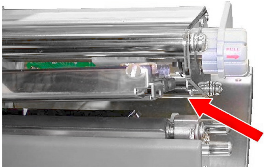
Abb. 9.2.1.d Druckkopf in seitliche Führungen einführen
