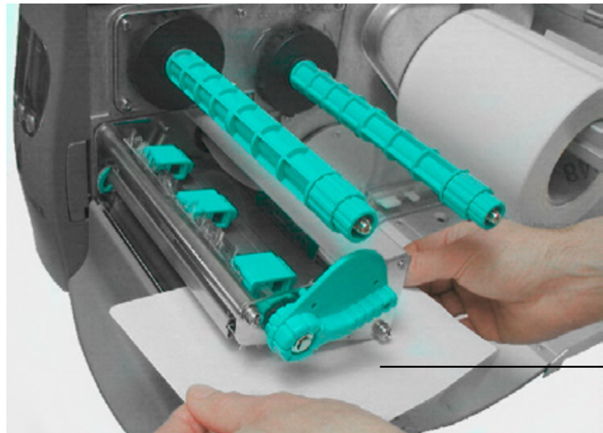
Abb. 9.1.2.b Druckkopf mit Reinigungsstreifen reinigen
