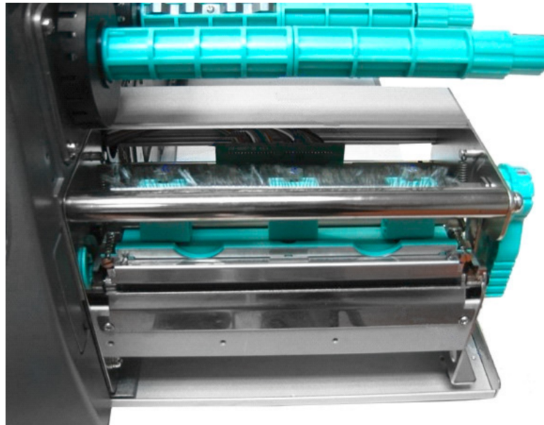
Abb. 5.4.f Druckkopf-Andruckkraft einstellen
