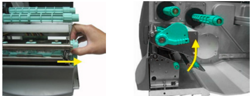
Abb. 9.2.1.a Druckkopf-Andruckhebel herausziehen und hoch schwenken (entgegen dem Uhrzeigersinn).
