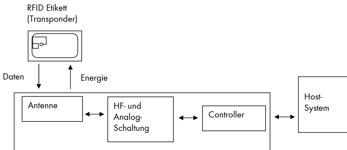
Abb. 1.2.a Blockdiagramm zur Hochfrequenz-Identifikationstechnologie (RFID)
