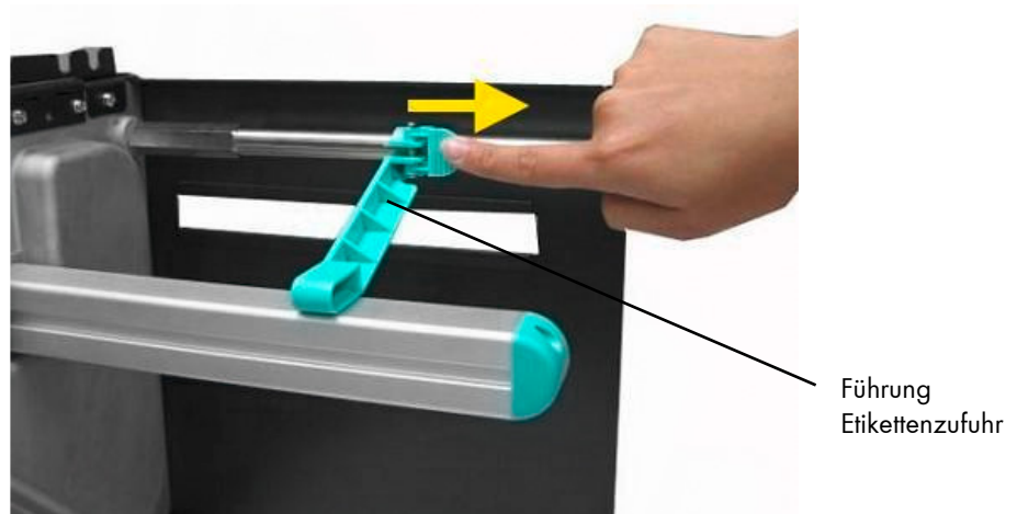
Abb. 5.2.1.c Führung Etikettenzufuhr nach rechts ziehen
