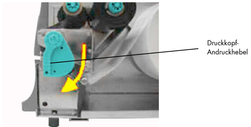
Abb. 5.4.e Andruckhebel schließen
