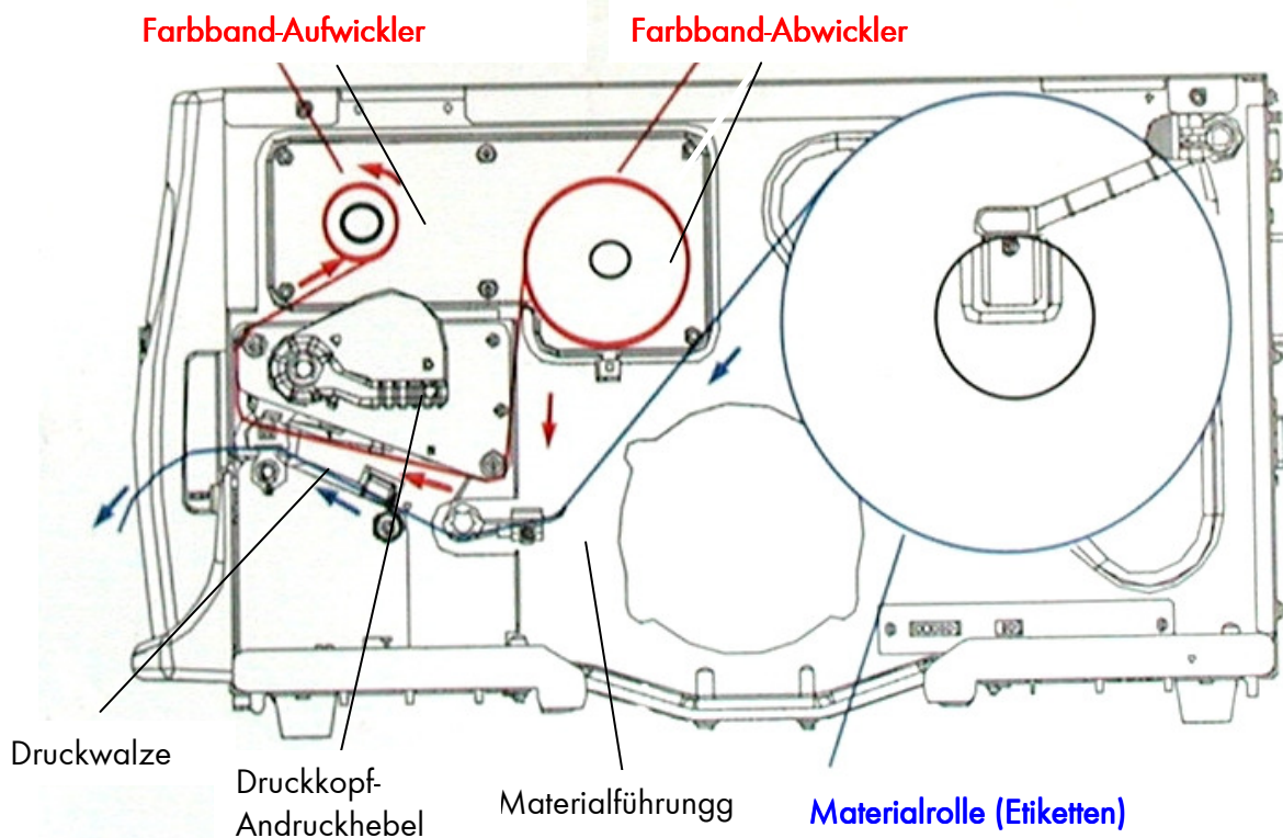
Abb. 5.1.a Material- und Folienverlauf (hier: Tinte auf der Innenseite der Rolle)
