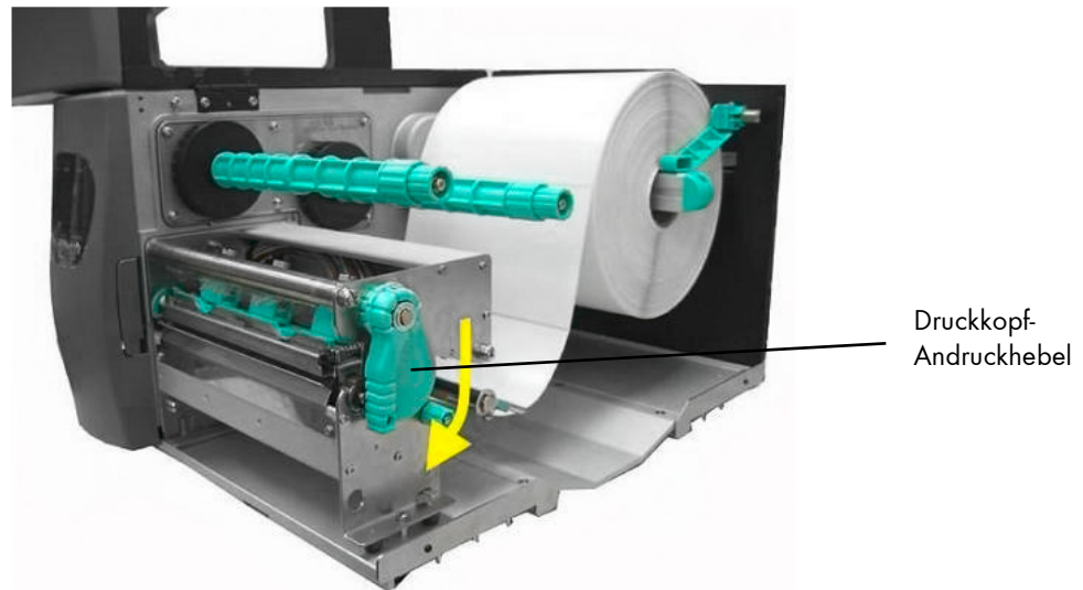
Abb. 5.2.1.m Andruckhebel schließen
