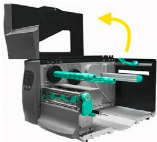
Abb. 5.2.1.b Haube des Druckers öffnen
