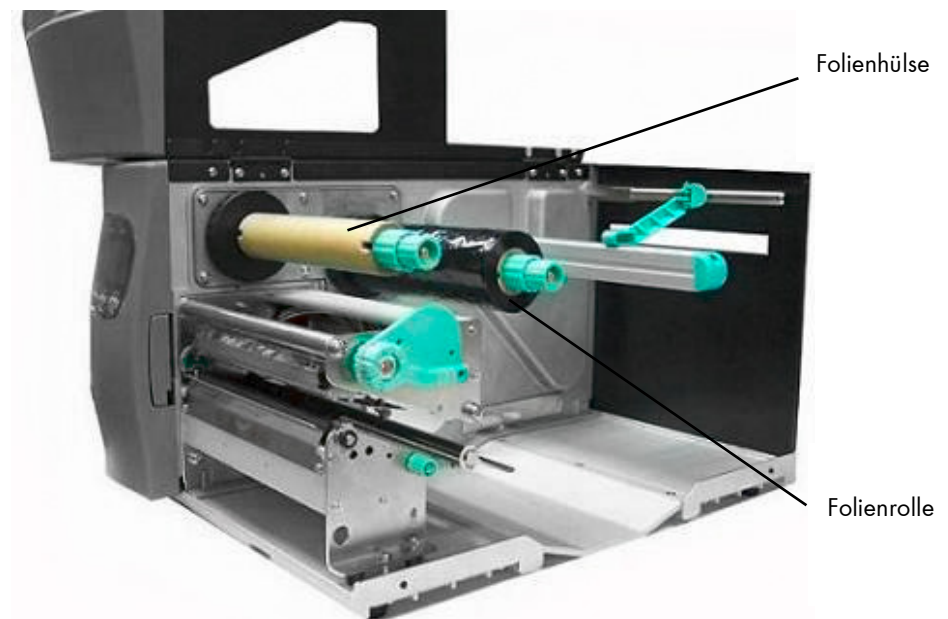
Abb. 5.3.1.c Folienrolle und leere Folienhülse einlegen
