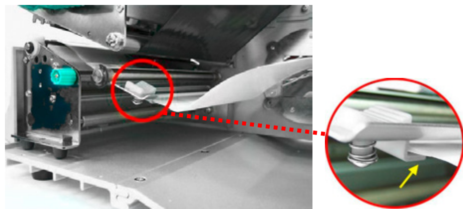
Abb. 5.2.1.j Materialführung einstellen
