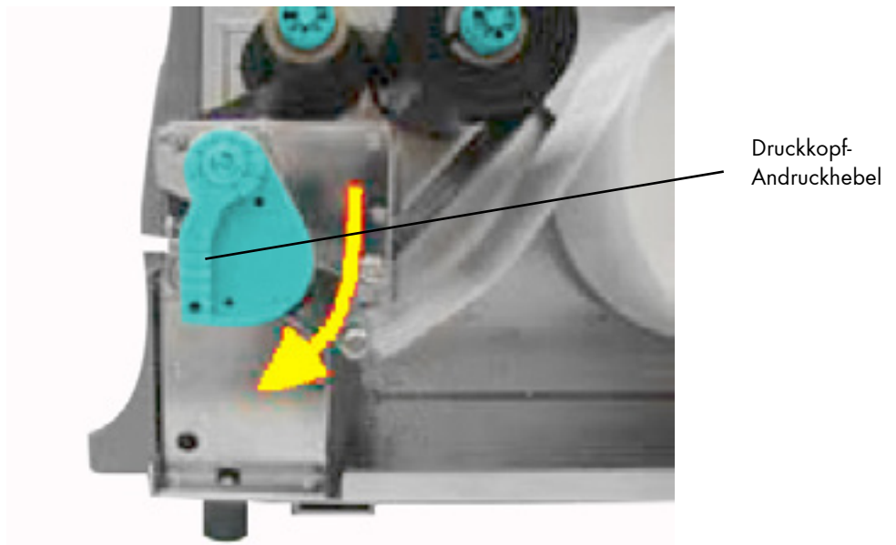
Abb. 5.3.1.f Andruckhebel verriegeln
