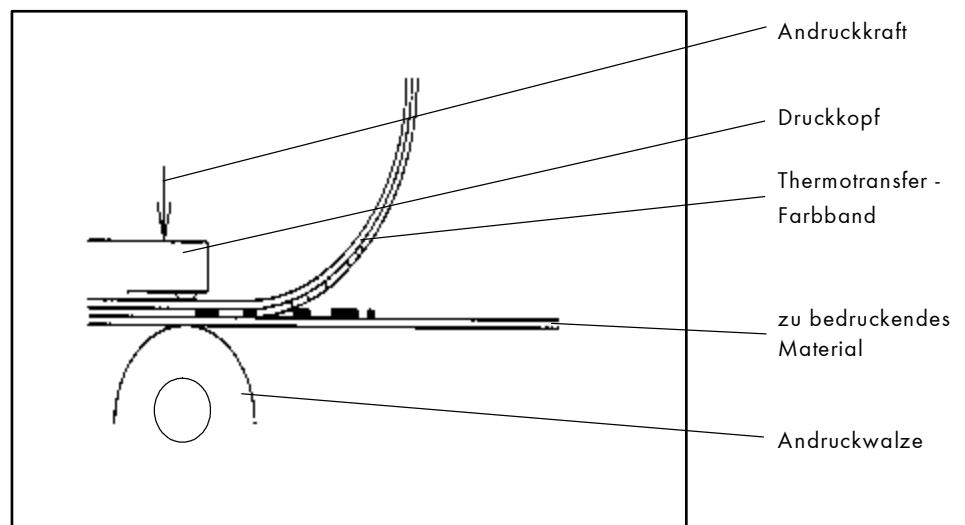
Abb. 9.3.a Schematische Darstellung des Druckprozesses
