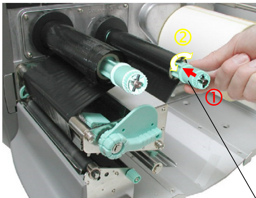
Abb. 5.3.2.a Farbbandspannung justieren
