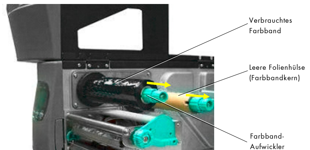
Abb. 5.3.3.a Verbrauchtes Farbband herausnehmen
