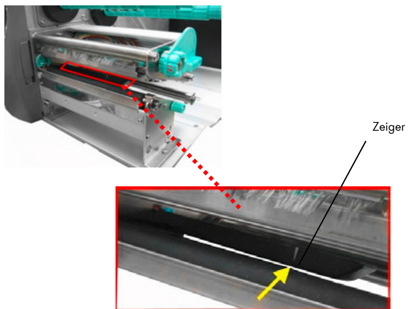
Abb. 5.2.1.l Der Zeiger zeigt die Sensorposition
