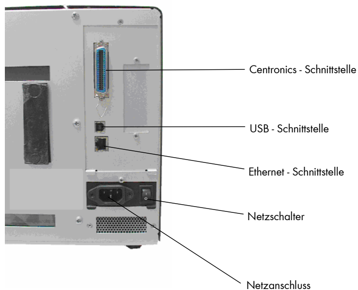
Abb. 2.4.b Rückansicht des Druckers
