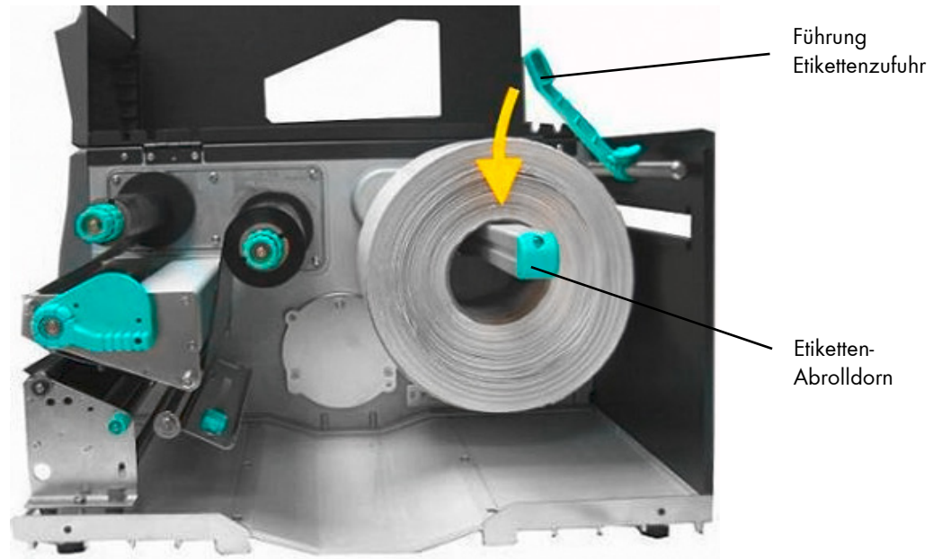
Abb. 5.2.1.e Materialrolle einlegen
