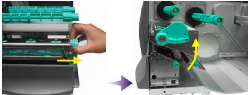
Abb. 5.4.b Druckkopf-Andruckhebel herausziehen und hoch schwenken (entgegen dem Uhrzeigersinn).
