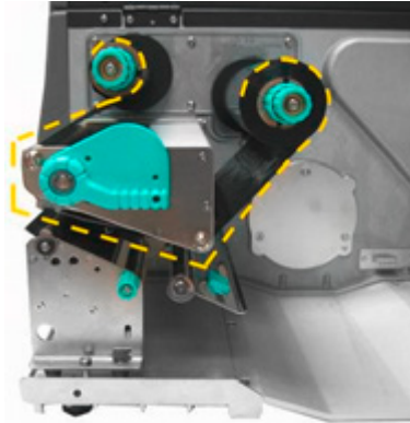
Abb. 5.3.1.b Unterschiedliche Wickelrichtungen für Folienrollen
