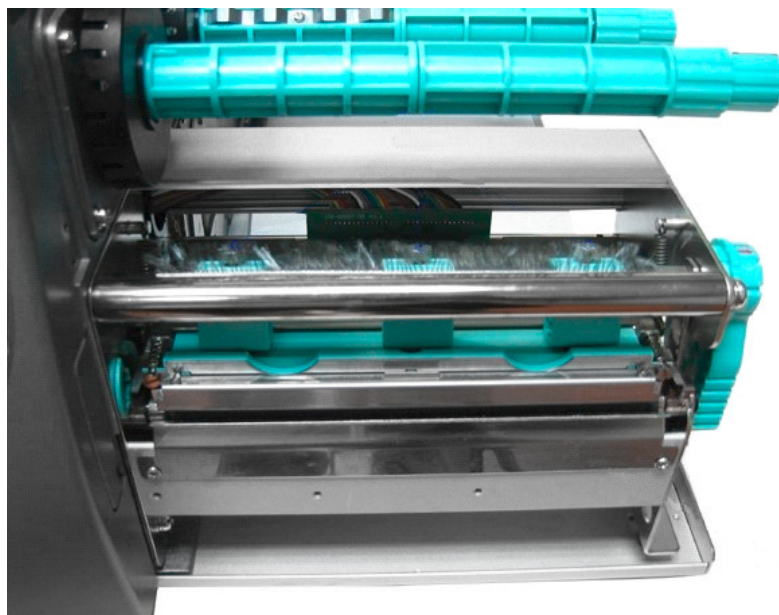
Abb. 5.4.a Druckkopf-Andruck: Position der Druckfederboxen
