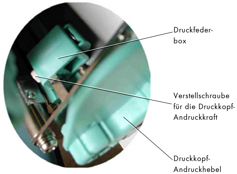
Abb. 5.4.d Detailaufnahme einer Druckfederbox
