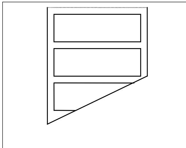
Abb. 5.2.1.a Abreiß-Rollenmaterial keilförmig zuschneiden
