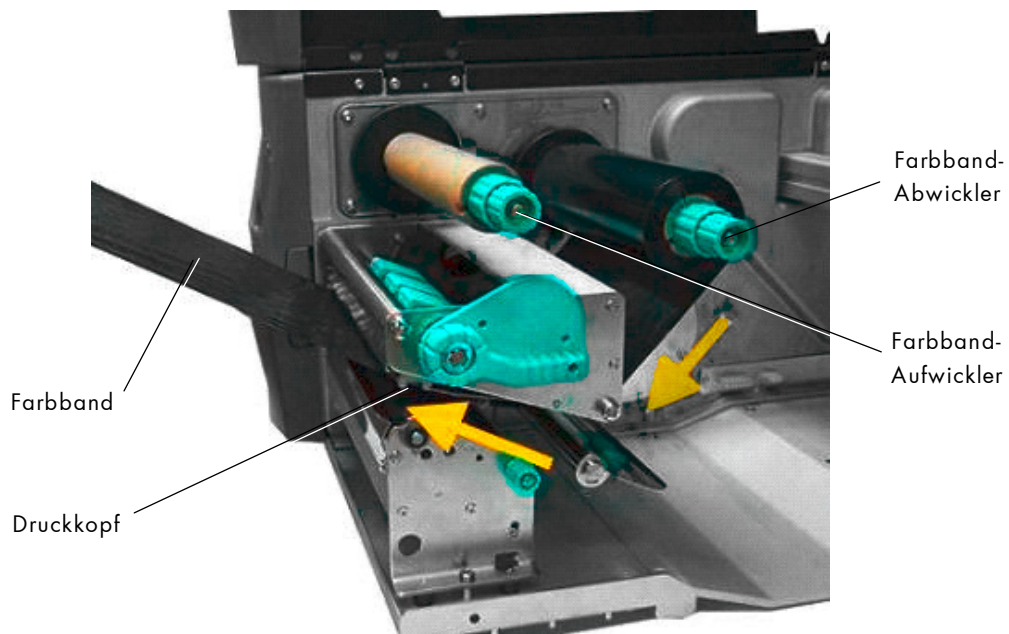
Abb. 5.3.1.d Folie unter Druckkopf hindurchführen
